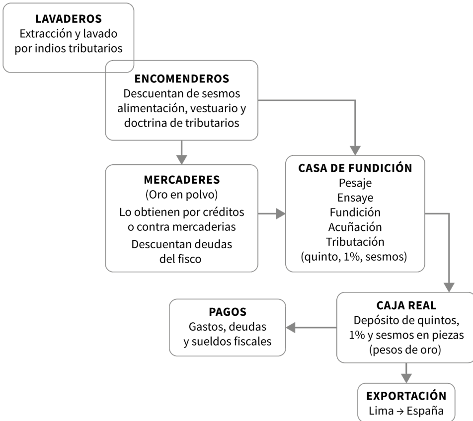
Figura 2. Circuito del oro de la Araucanía, siglo XVI
